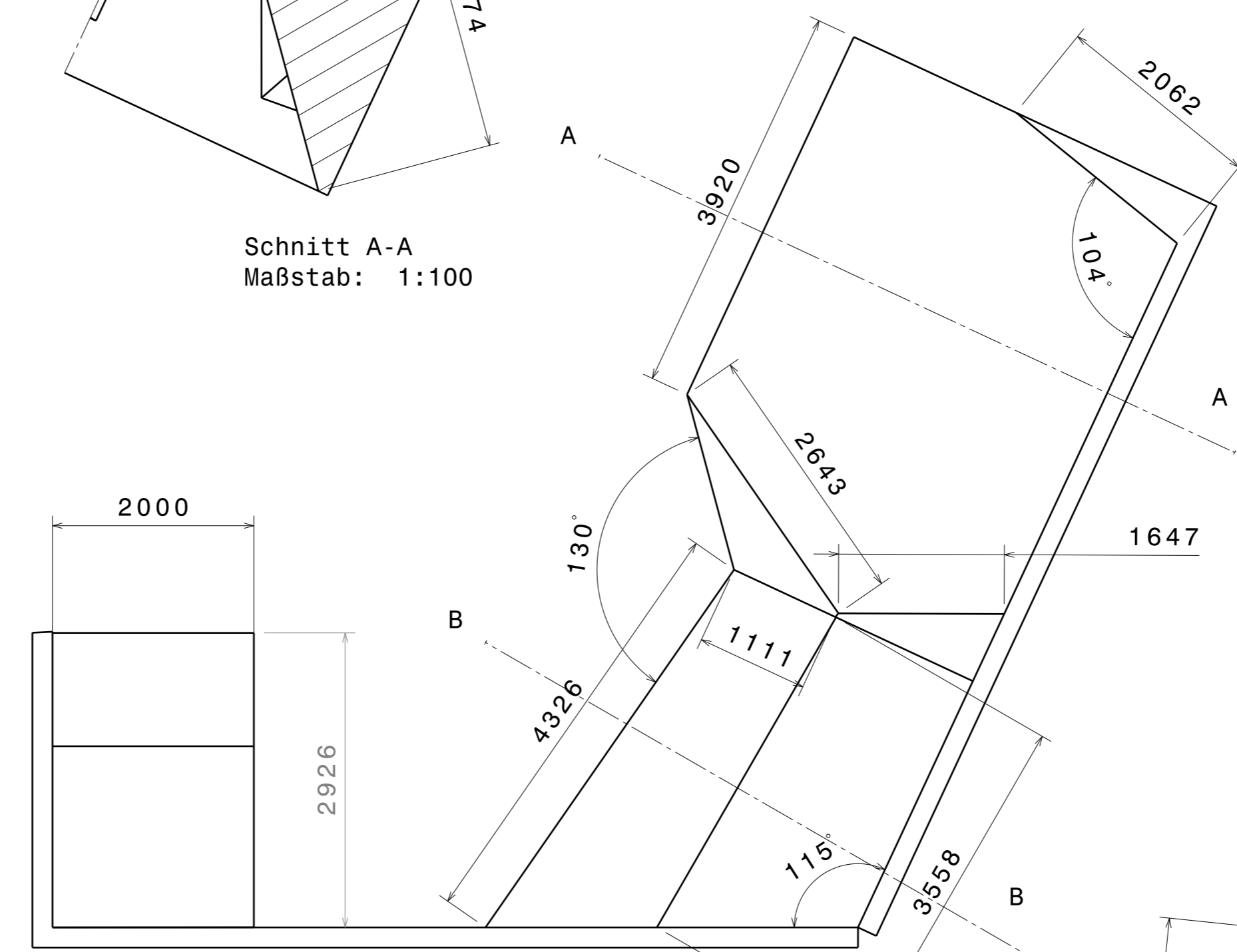
Unten Maßstab: 1:50
