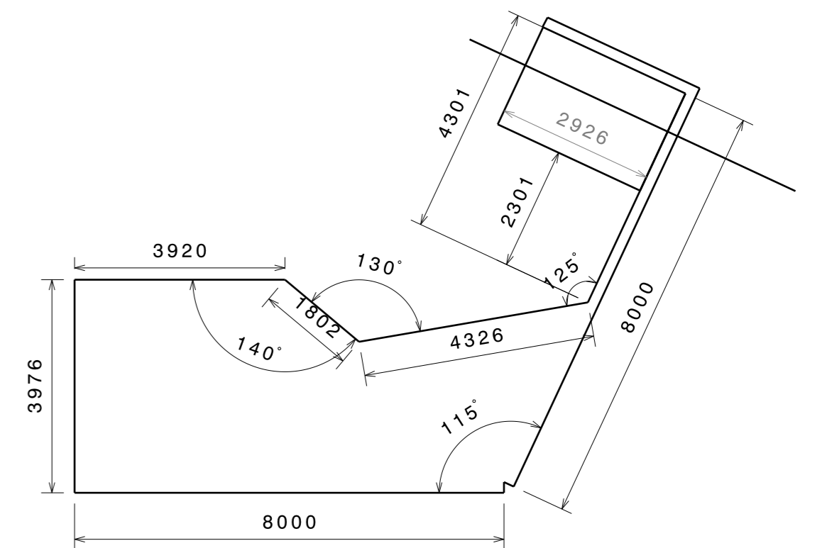
Oben Maßstab: 1:100
