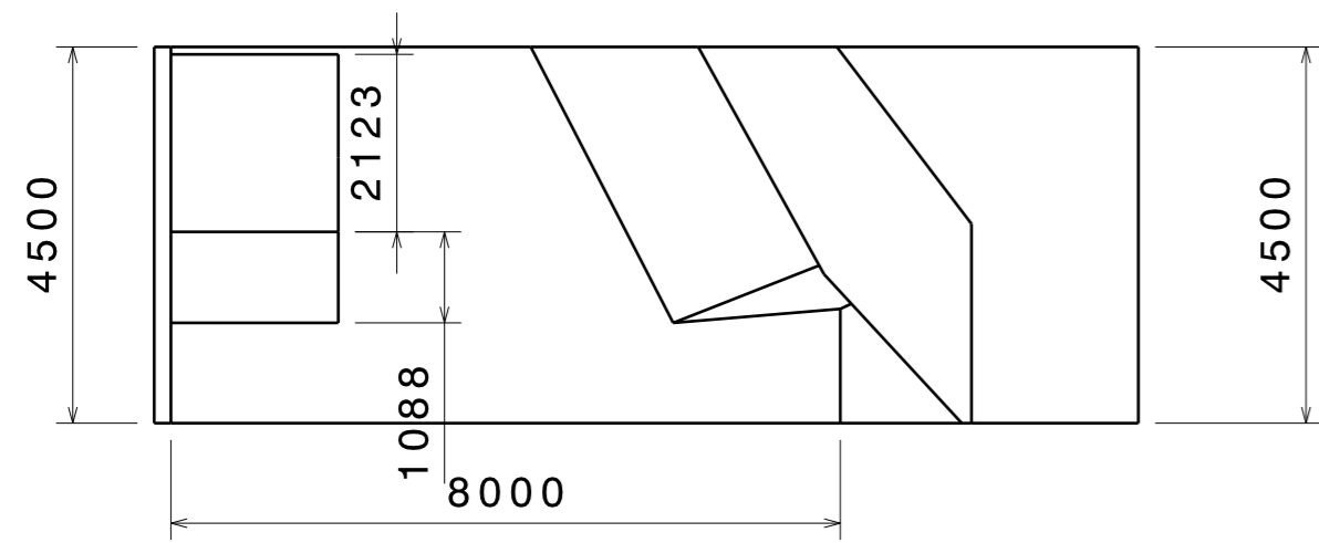
Seite Maßstab: 1:100
