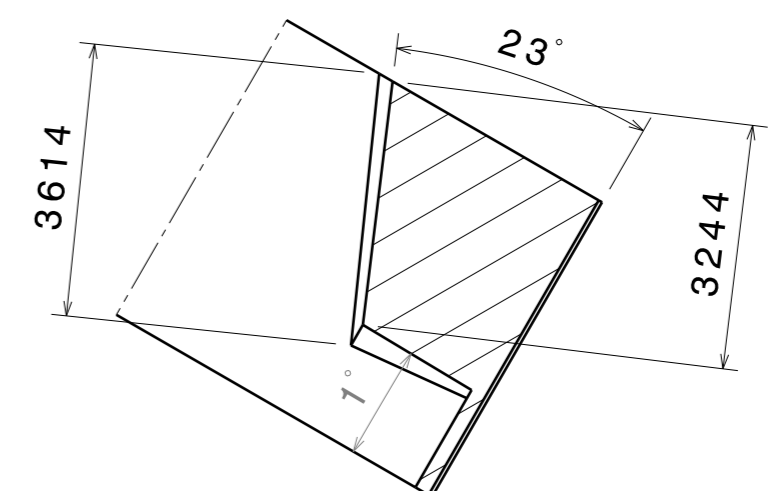
Schnitt B-B Maßstab: 1:100
